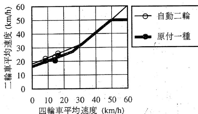
図12-1 四輪車の速度と二輪車の速度の関係
