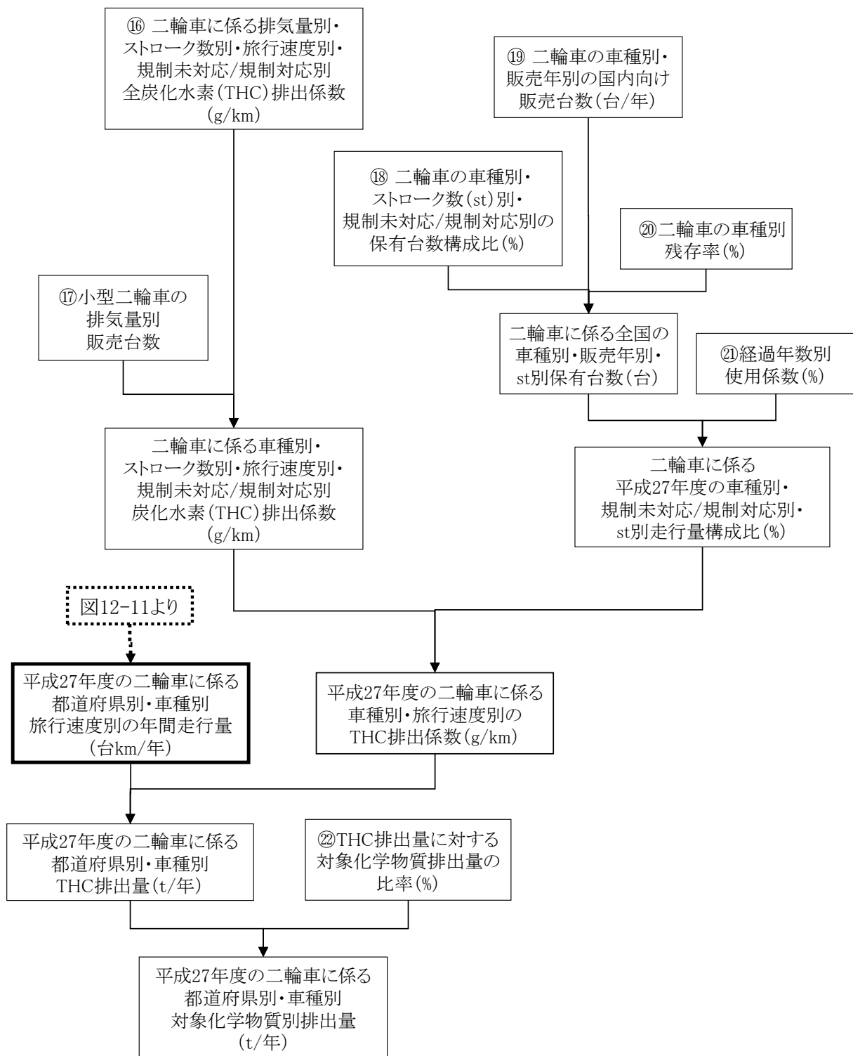
図12-9 二輪車(ホットスタート)に係る対象化学物質別排出量の推計フロー
