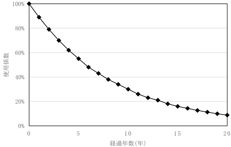
図12-6 経過年数ごとの使用係数
