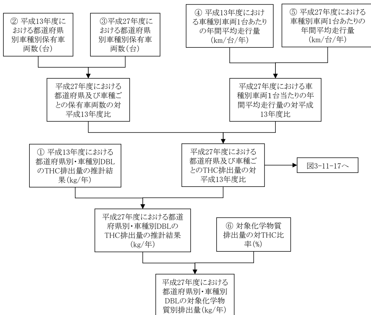
図12-12 燃料蒸発ガス(DBL)に係る推計フロー
