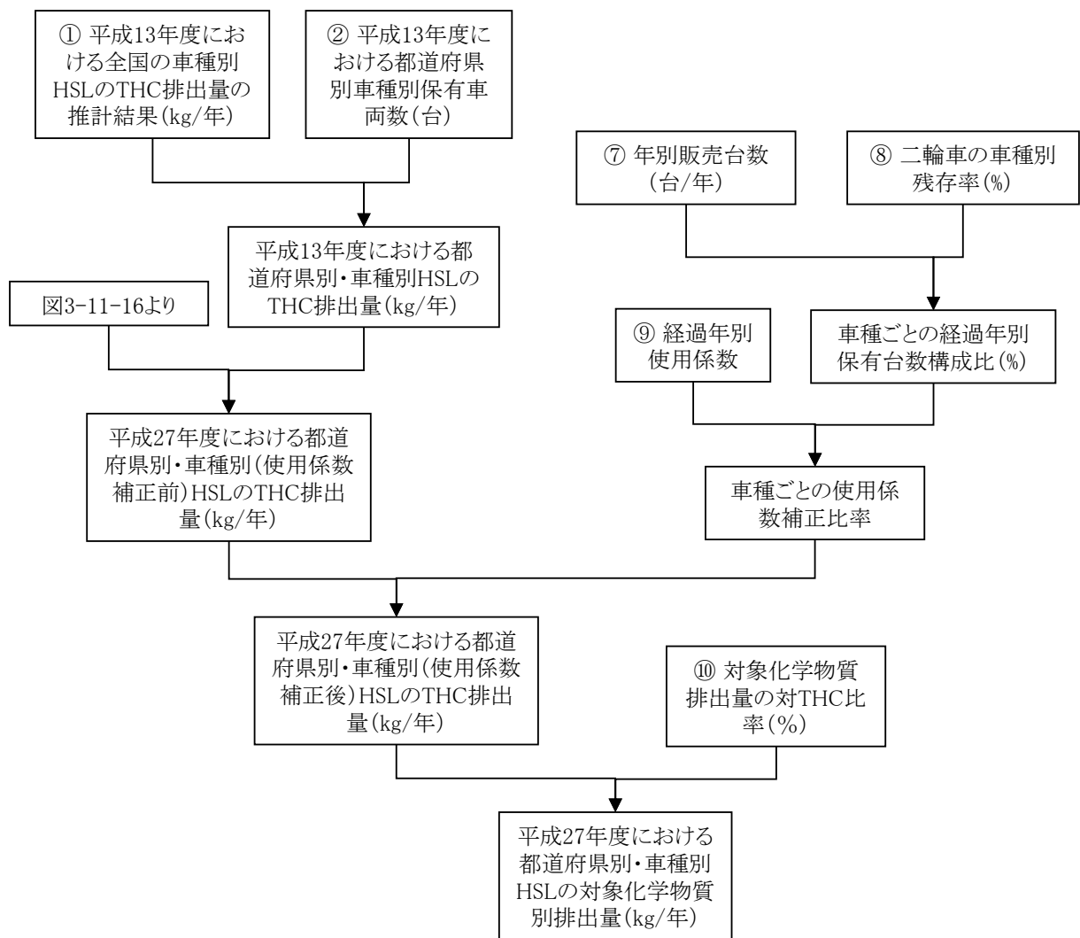
図12-13 燃料蒸発ガス(HSL)に係る推計フロー
