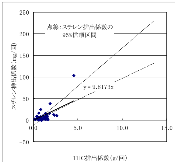
図12-15 二輪車(コールドスタート時の増分)に係る THC 排出量と対象化学物質別排出量の比率(その1)
