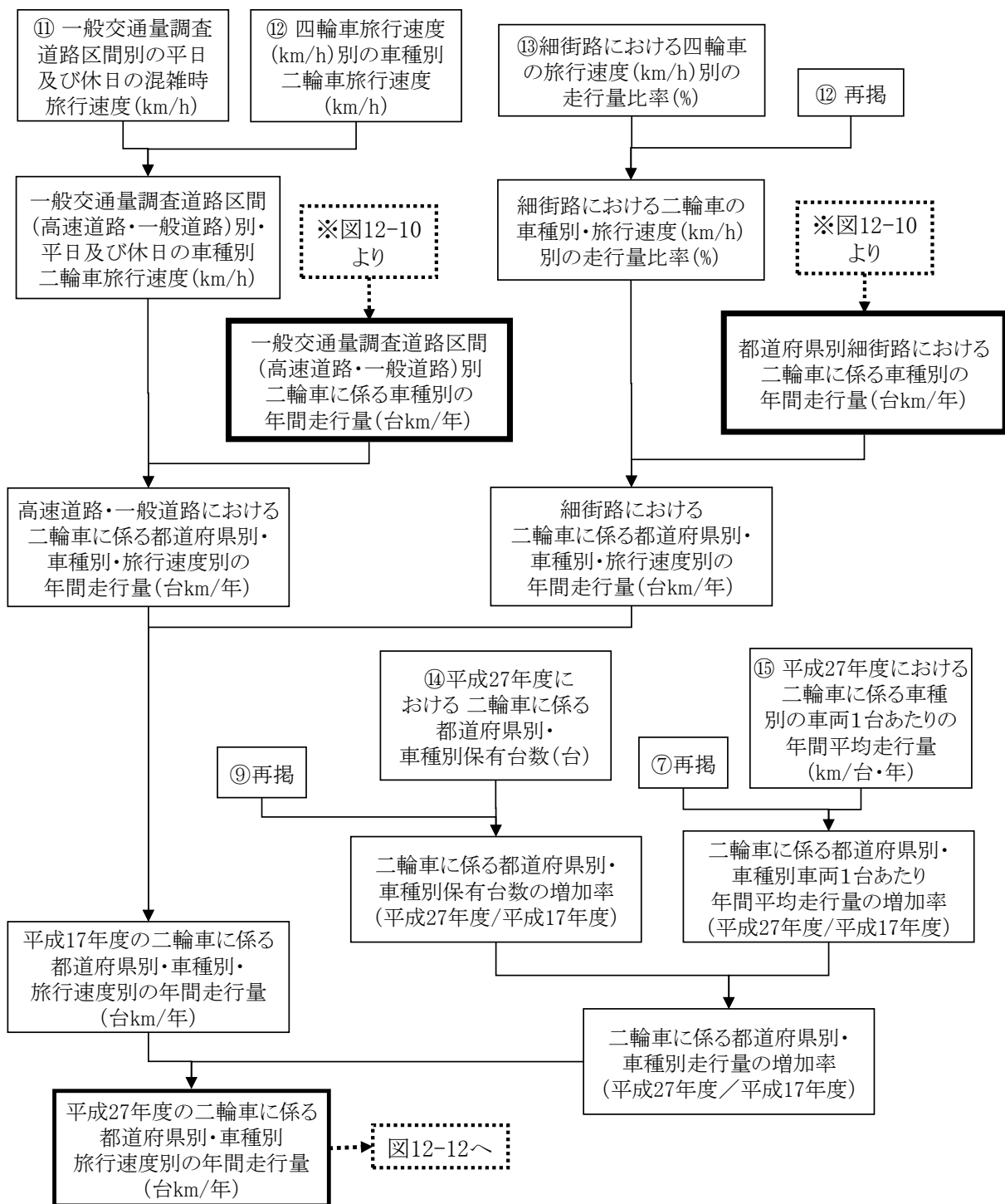
図12-8 二輪車の都道府県別・車種別年間走行量の推計フロー
