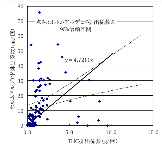
図12-15 二輪車(コールドスタート時の増分)に係る THC 排出量と対象化学物質別排出量の比率(その2)
