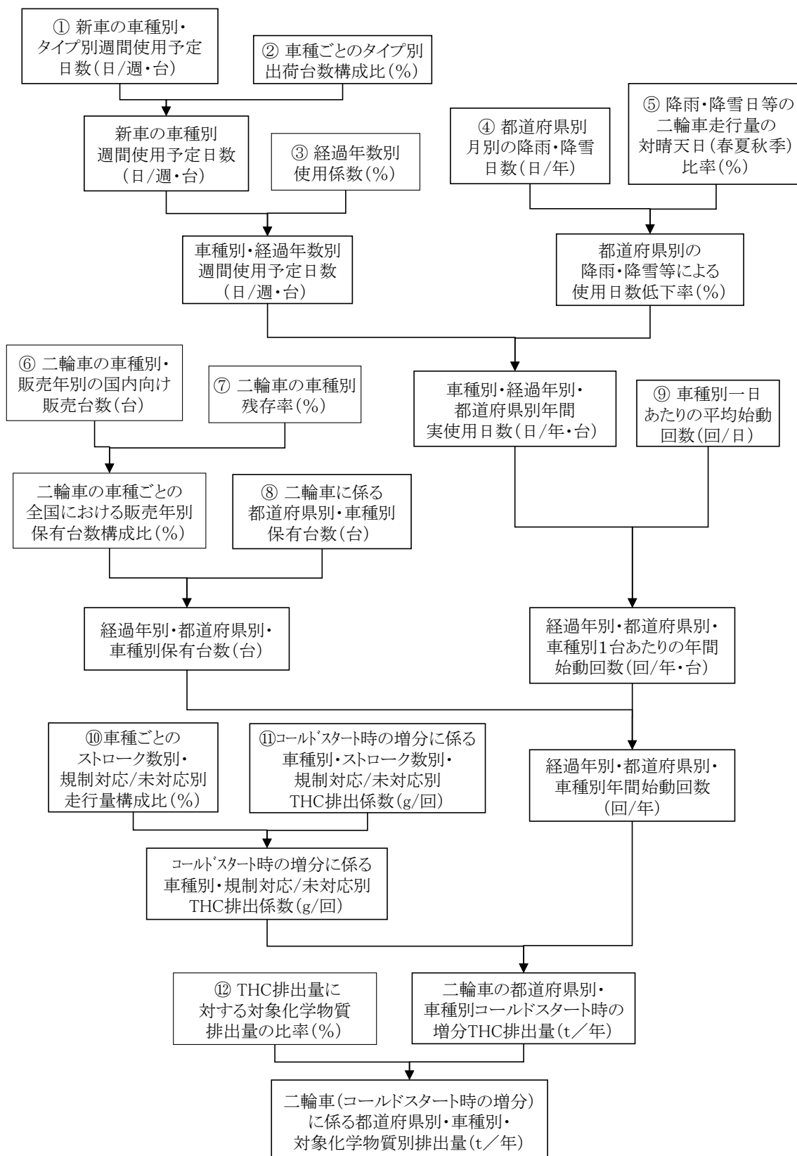
図12-11 二輪車(コールドスタート時の増分)に係る排出量推計フロー
