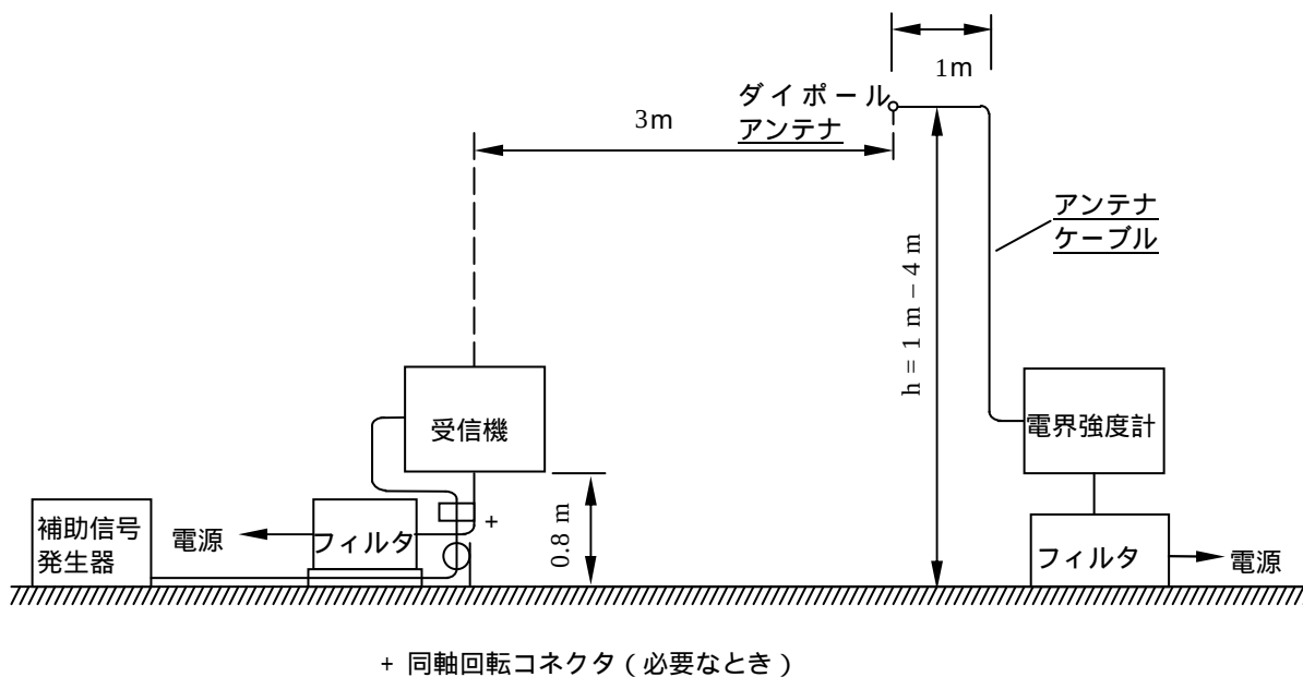
図 14 3 m の距離における屋外電界測定 (5.7.3 項参照)
