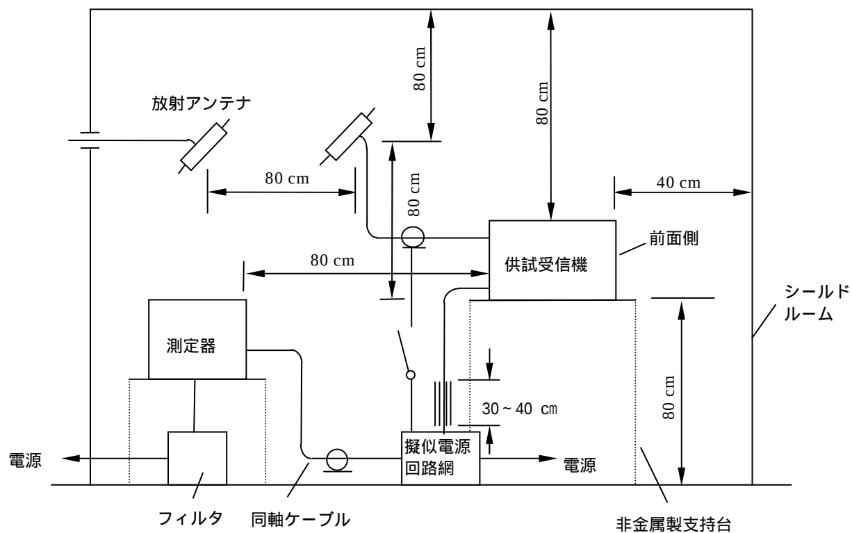
図5 電源端子妨害波電圧測定（5.3.1 項参照）
