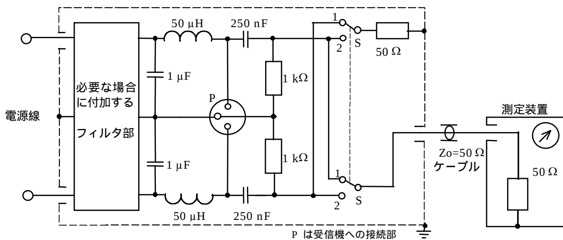
図3 50 \Omega - 50 \mu H の擬似電源回路網の例 ( 5.3.1 項参照 )
