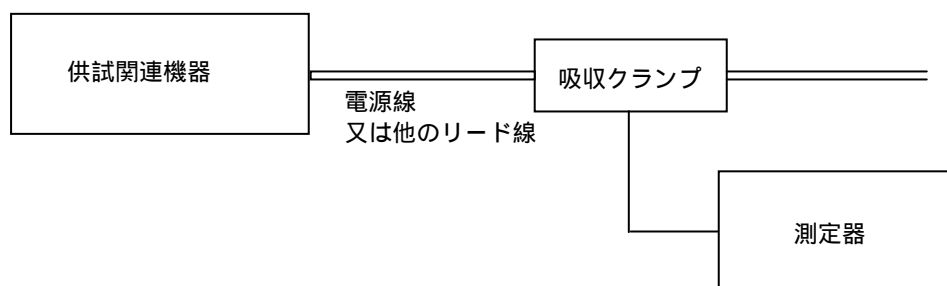
図 10 関連機器（チューナをもつビデオレコーダを除く）の 妨害波電力測定のための回路構成（5.6.3 項参照）
