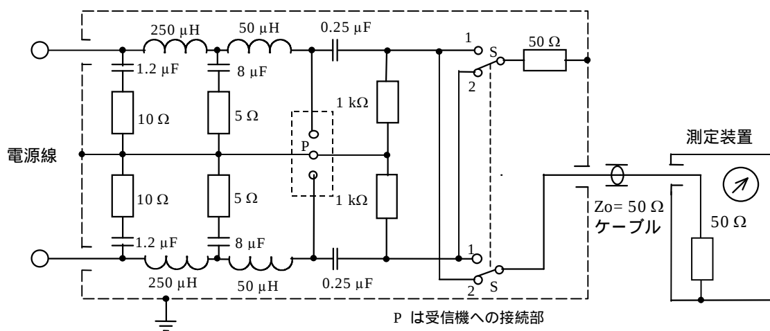
図4 50 \Omega - 50 \mu H - 5 \Omega の擬似電源回路網の例 ( 5.3.1 項参照 )
