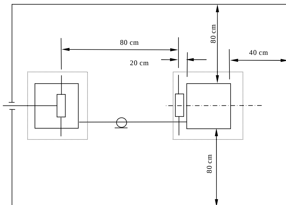
図6 電源端子妨害波電圧測定（配置-平面図） （5.3.1 項参照）
