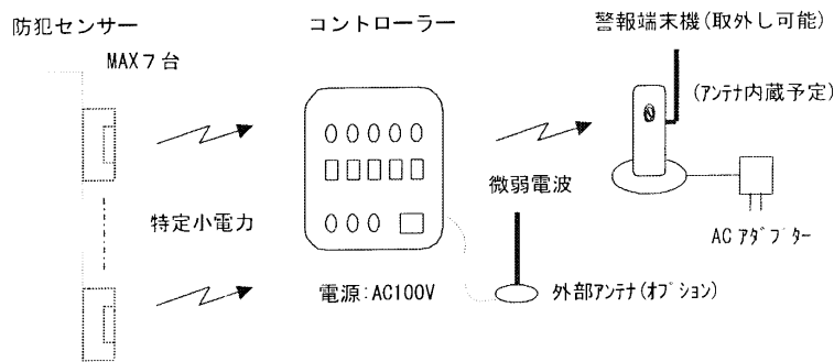
概略構成図
