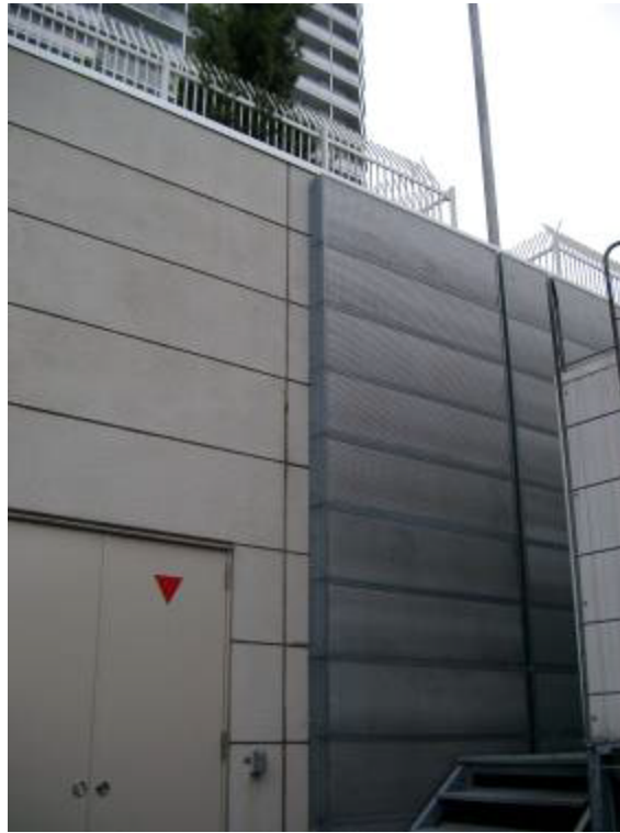
冷却塔横に設置した吸音板
