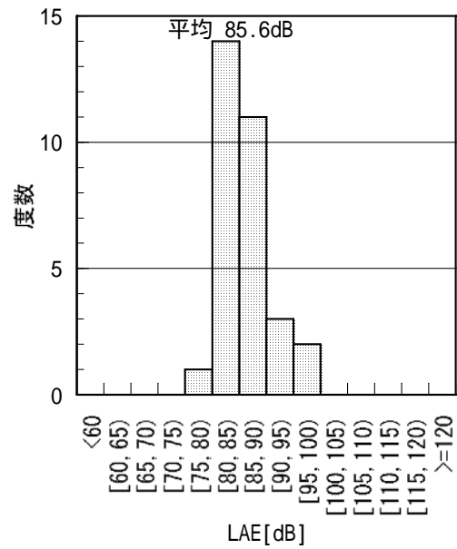
(4) L_{AE}
