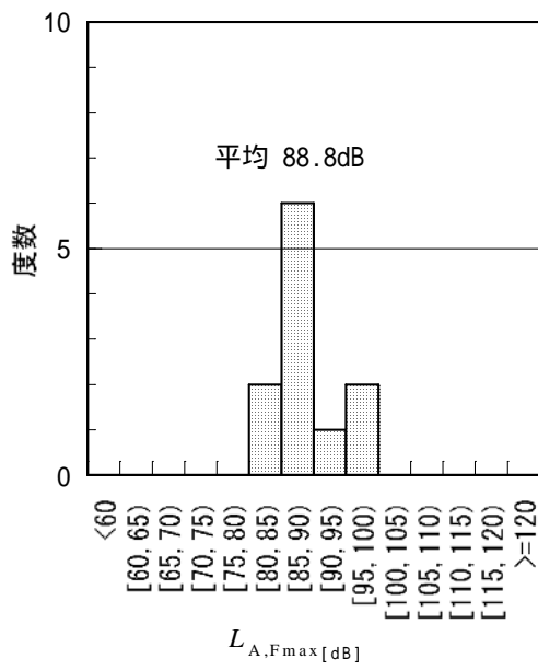
(3) L_{A,Fmax}
