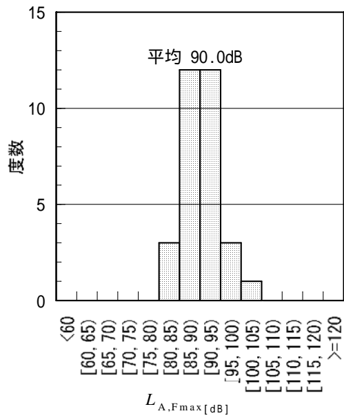
(3) L_{A,Fmax}
