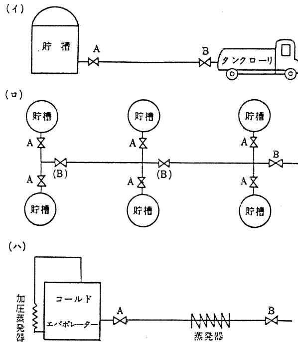
A; 貯槽の直近に設けたバルブ B; 他の一つのバルブ (B); 必ずしも設けなくともよいバルブ
