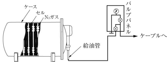
ガス封じ込め型（外ガス型）（セルの内部に絶縁油を充てんしケース本体にN 2 ガスを封入したもの）
