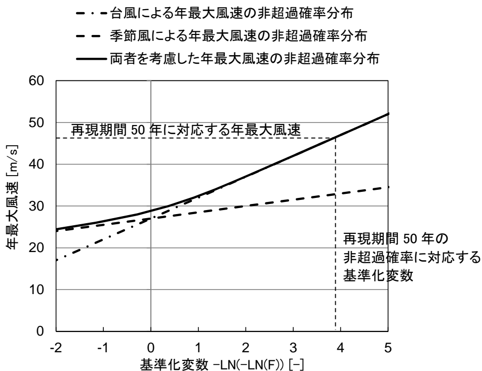
図-解 3.1.5 混合非超過確率分布の例
