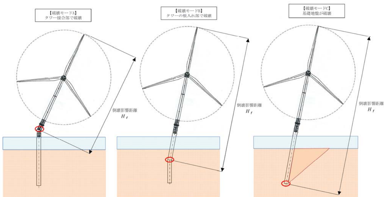
図-解 2.7.1 杭式基礎の破壊モードの参考例 1)
