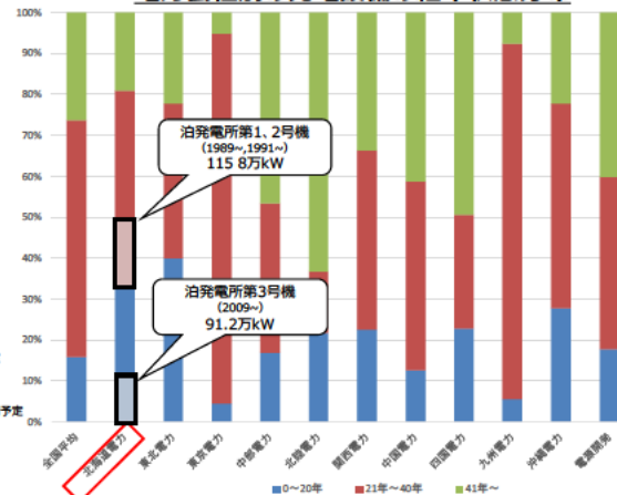
電力会社別の発電設備の経年状態分布
