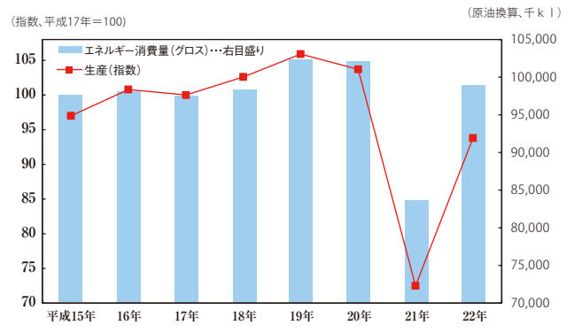
鉄鋼業の生産とエネルギー消費量の推移
