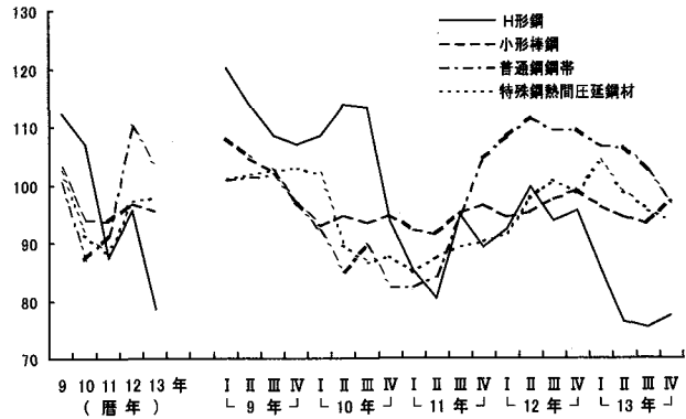
第5図 熱間圧延鋼材の主要品目の生産推移 (7年=100、季節調整済)
