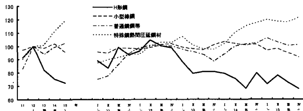
第2-4図 熱間圧延鋼材の主要品目の生産推移 (平成12年=100、季節調整済)
