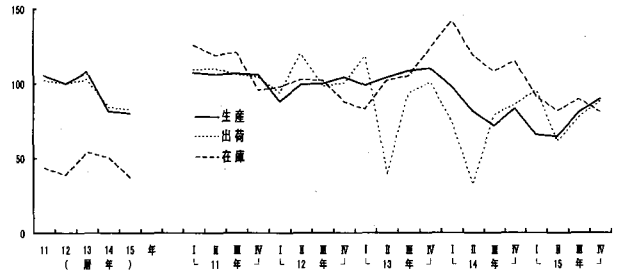
第4-5図 石油ストーブの生産・出荷・在庫の推移 (平成12年=100、季節調整済)
