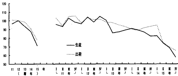
第4-3図 橋りょうの生産・出荷の推移 (平成12年=100、季節調整済)
