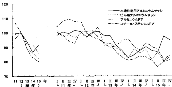
第4-4図 建築用金属製品の生産の推移 (平成12年=100、季節調整済)
