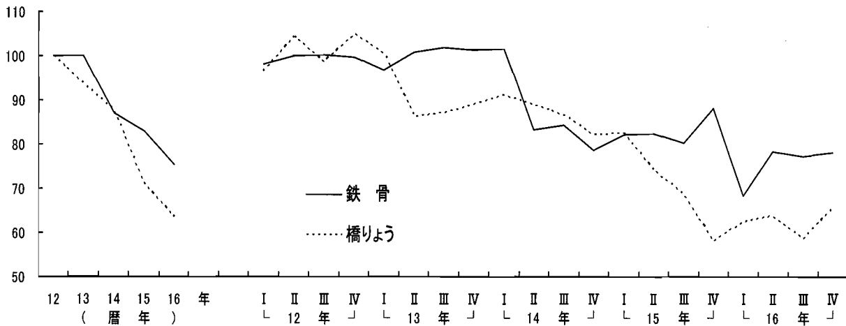
第4-4図 建築用金属製品の生産の推移 (12年=100、季節調整済)
