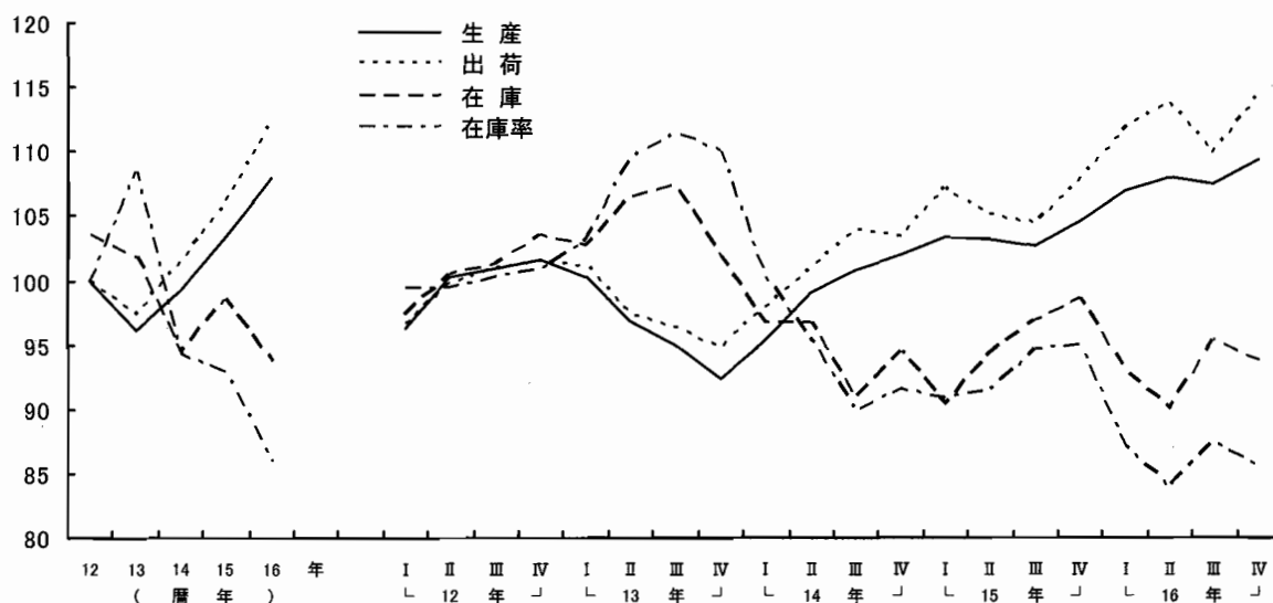
第2-1図 鉄鋼業指数の推移 (12年=100、季節調整済)
