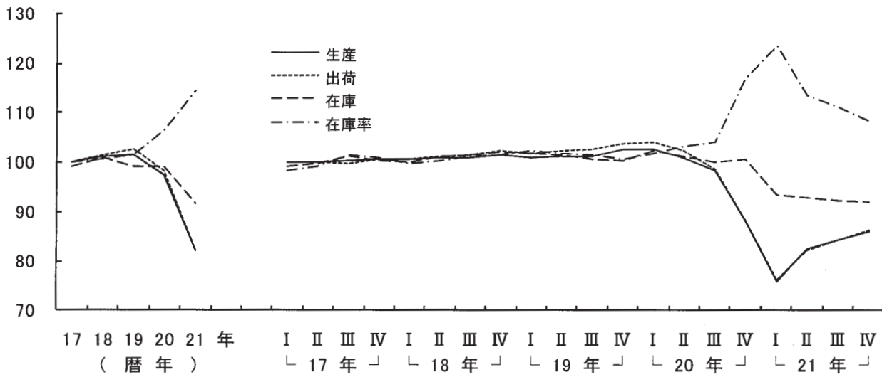
第9図 プラスチック製品工業の生産、出荷、在庫及び在庫率の推移 (17年=100、季節調整済)
