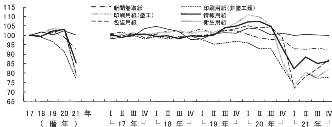
第5図 紙の品目別生産の推移
