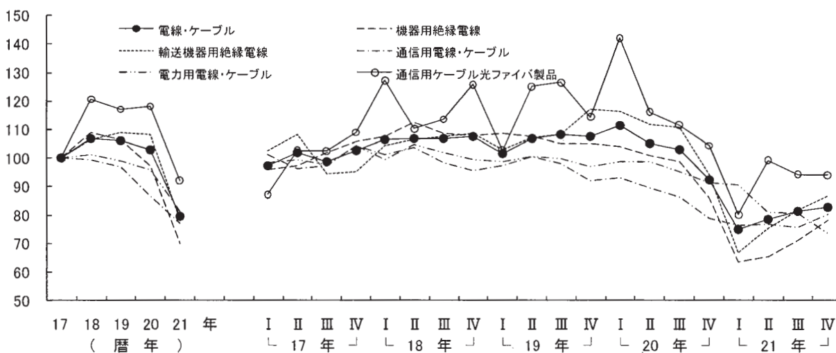
第3-5図 電線・ケーブルの生産の推移
