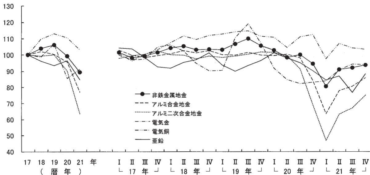
第3-3図 非鉄金属地金の生産の推移
