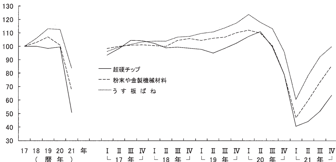
第4-6図 超硬チップ、粉末や金製機械材料、うす板ばねの生産の推移
