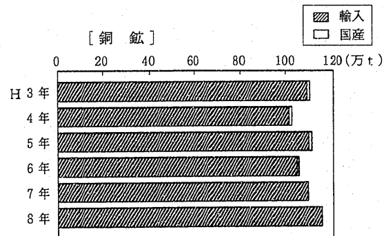
第4図 銅鉱・鉛鉱・亜鉛鉱の国内生産と輸入の推移
