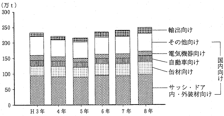
第14図 アルミニウム圧延製品の用途別推移
