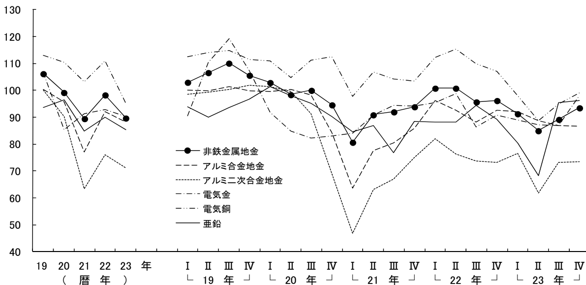
第3-3図 非鉄金属地金の生産の推移
