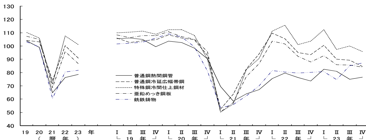
第2-5図 鉄鋼主要品目の生産の推移
