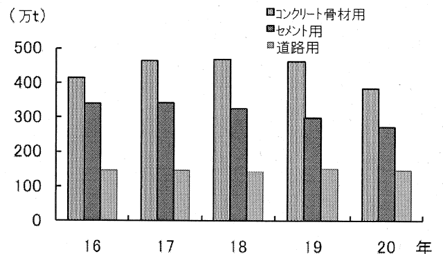
第9図 けい石の主要販売内訳
