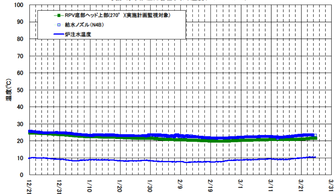
2号機 原子炉圧力容器まわり温度(12/21~3/25)
