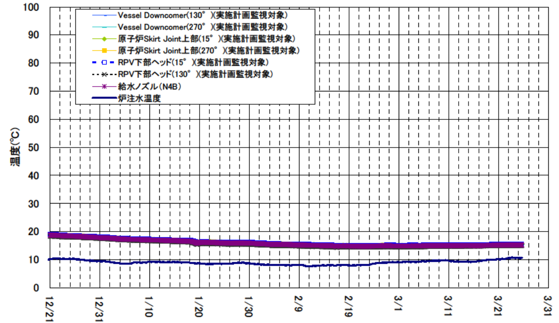
1号機 原子炉圧力容器まわり温度 (12/21~3/25)
