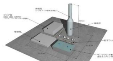
③ 水蒸気放出の例
