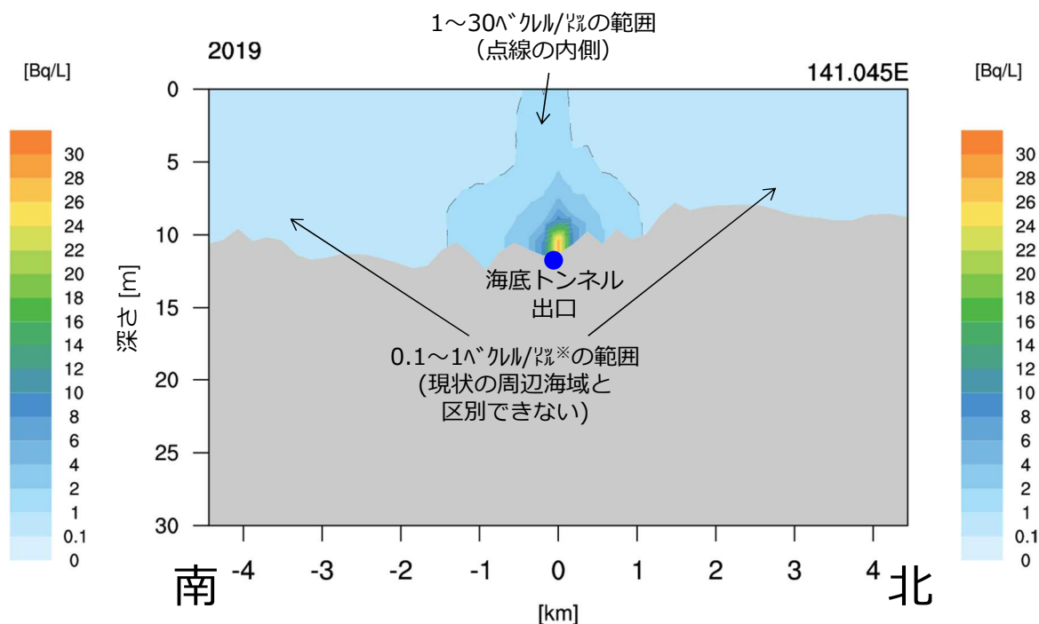
トンネル出口南北断面図 （最大目盛30ベクレル/ℓにて作図）
