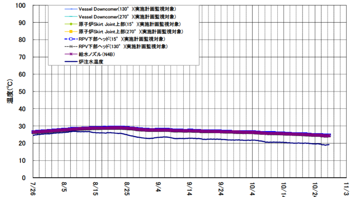
1号機 原子炉圧力容器まわり温度(7/26~10/28)
