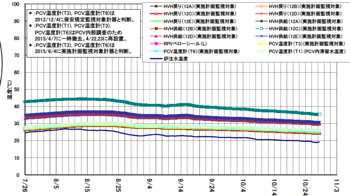
1号機 D/W雰囲気温度(7/26~10/28)
