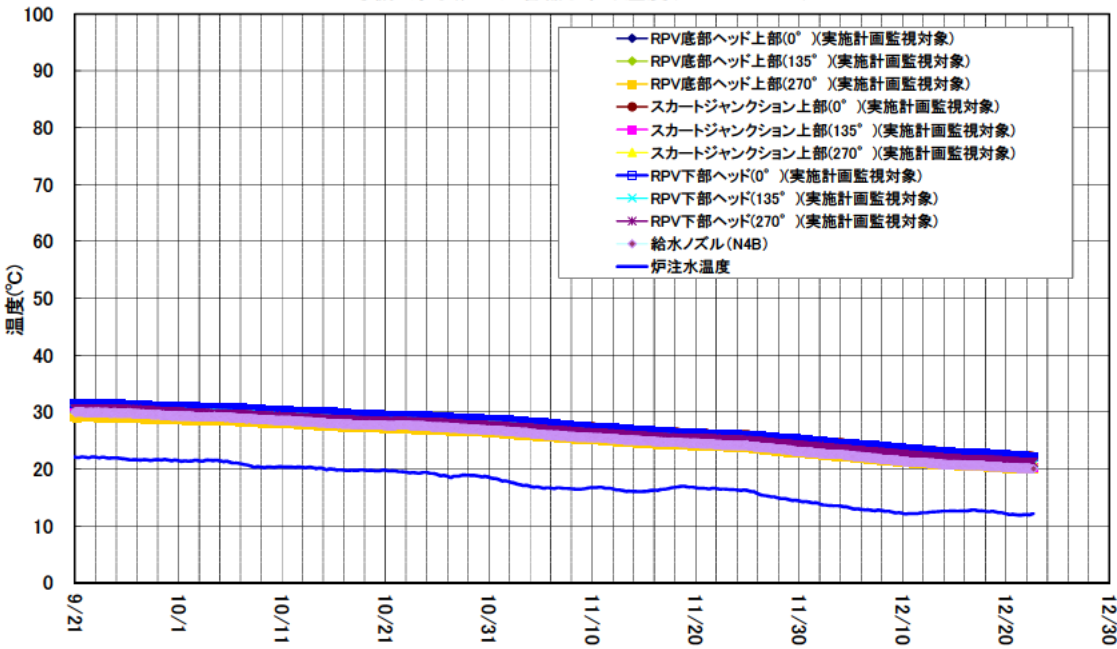
3号機 原子炉圧力容器まわり温度(9/21～12/22)
