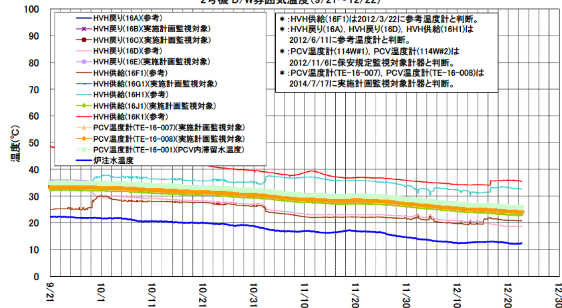
2号機 D/W雰囲気温度(9/21~12/22)
