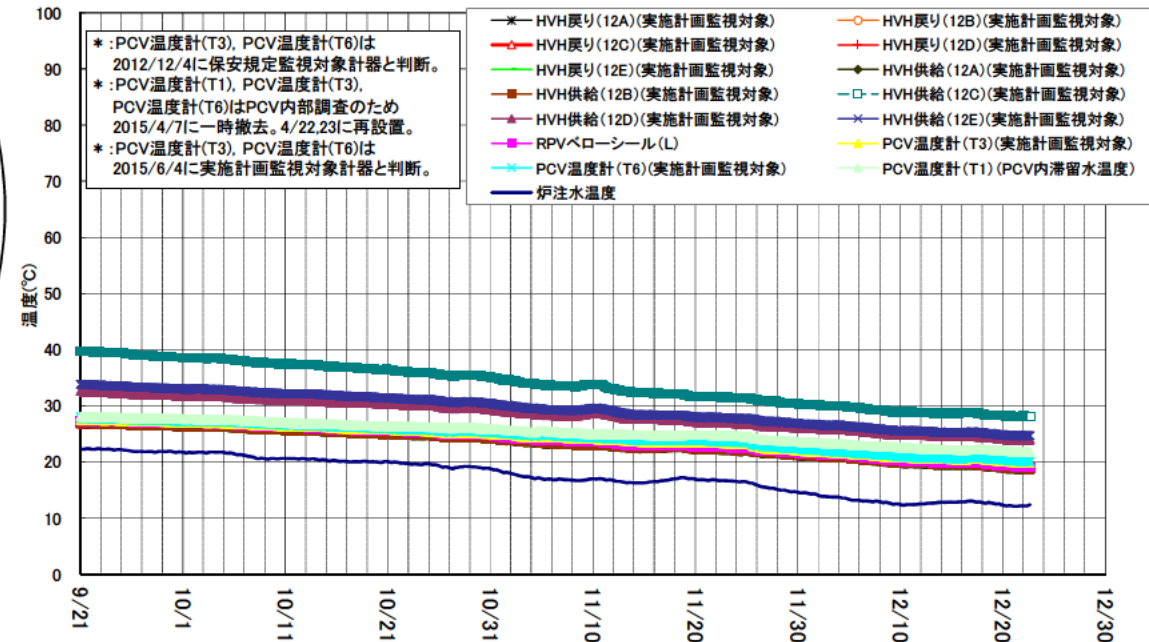
1号機 D/W雰囲気温度(9/21~12/22)
