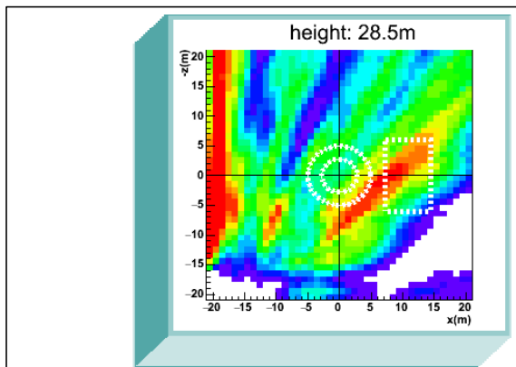
測定装置1
