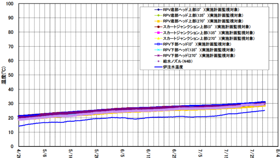
3号機 原子炉圧力容器まわり温度(4/26～7/29)
