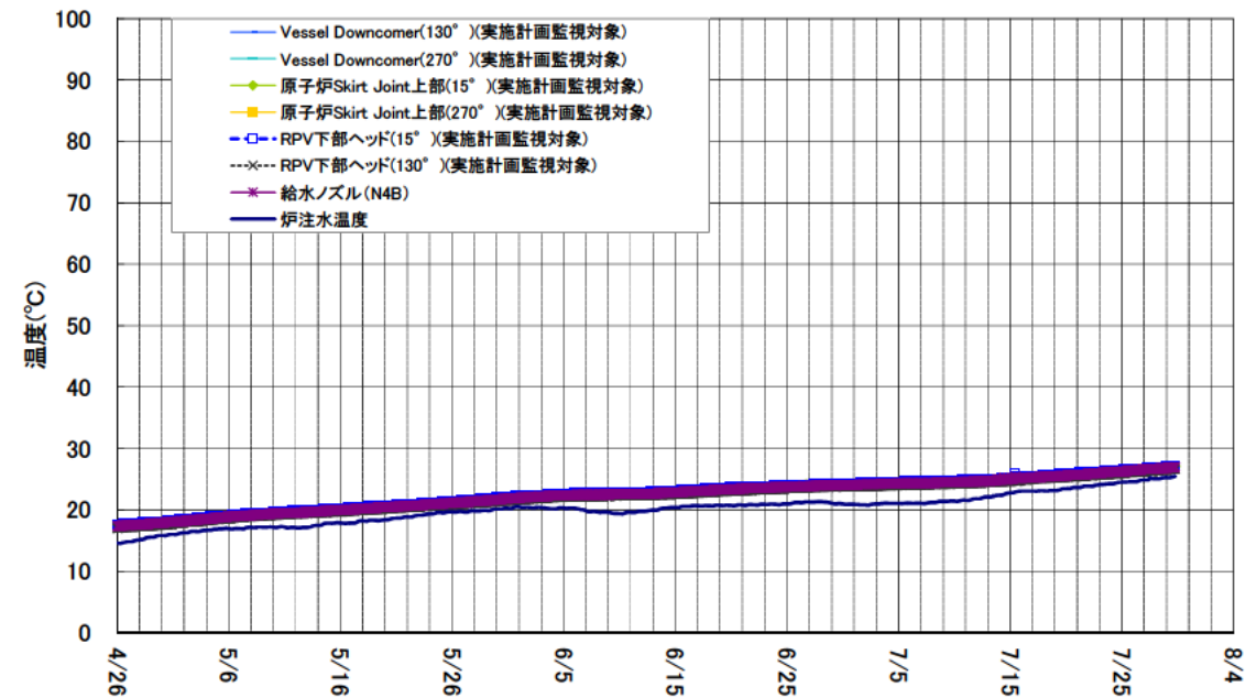
1号機 原子炉圧力容器まわり温度(4/26~7/29)
