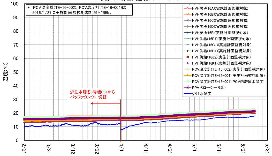
3号機 D/W雰囲気温度 (2/21~5/25)
