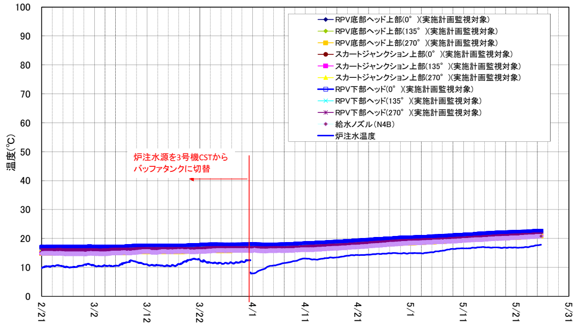
3号機 原子炉压力容器まわり温度 (2/21~5/25)
