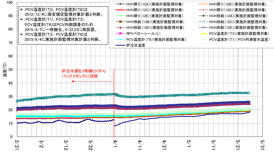
1号機 D/W雰囲気温度(2/21~5/25)
