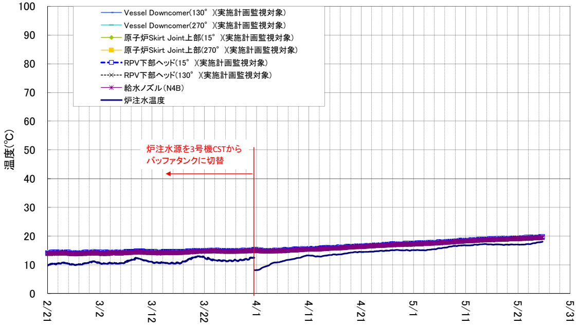
1号機 原子炉压力容器まわり温度(2/21~5/25)
