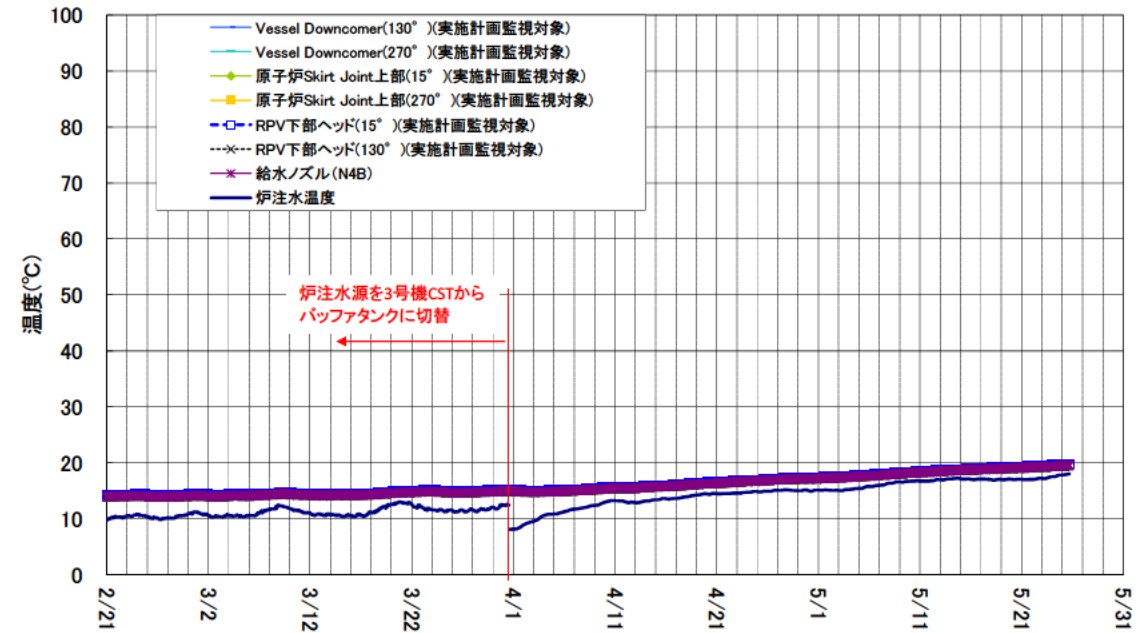
1号機 原子炉圧力容器まわり温度(2/21~5/25)
