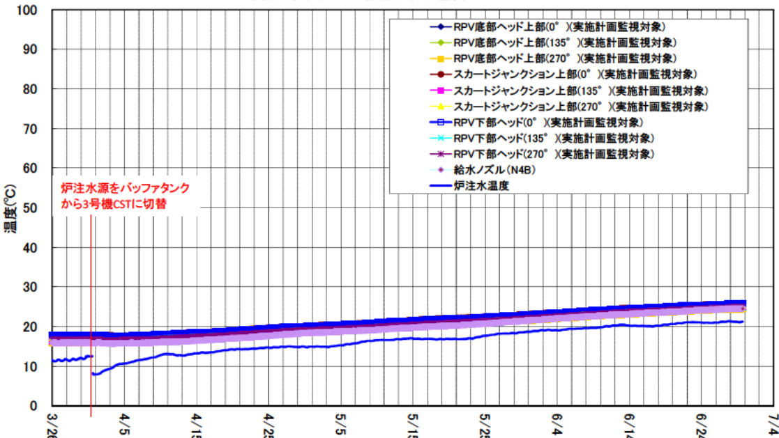
3号機 原子炉圧力容器まわり温度(3/26～6/29)
