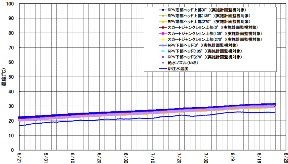
3号機 原子炉圧力容器まわり温度(5/21～8/24)
