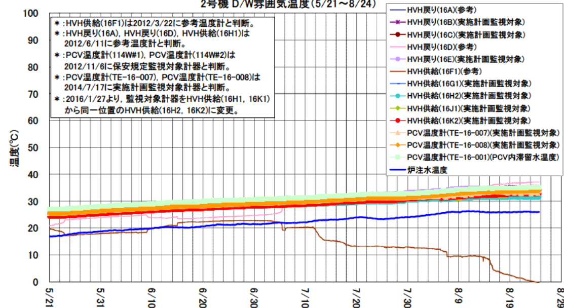
2号機 D/W雰囲気温度(5/21~8/24)
