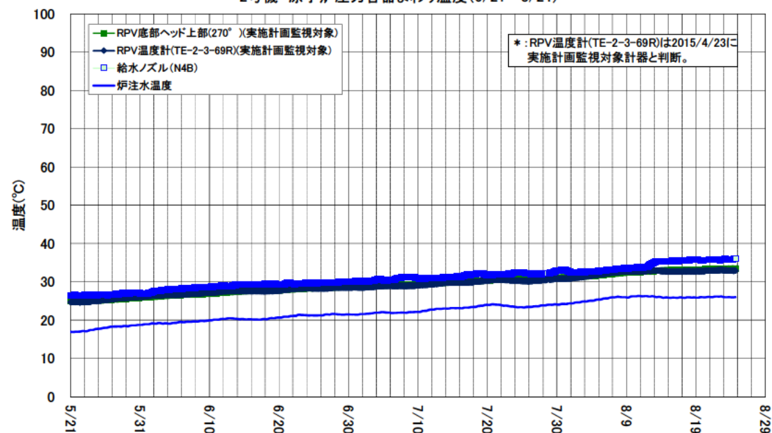
2号機 原子炉压力容器まわり温度(5/21~8/24)
