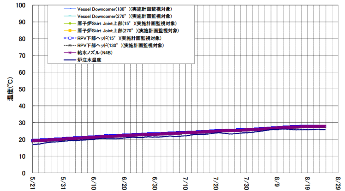
1号機 原子炉圧力容器まわり温度(5/21~8/24)
