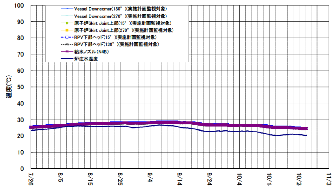
1号機 原子炉圧力容器まわり温度(7/26~10/26)
