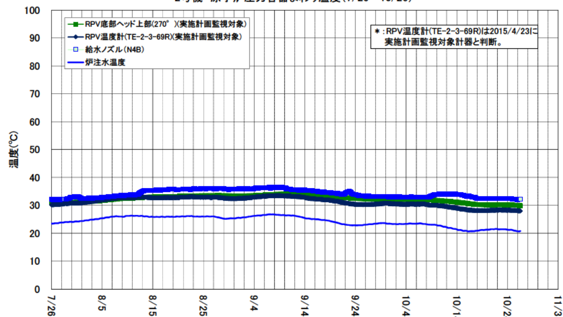
2号機 原子炉压力容器まわり温度(7/26~10/26)
