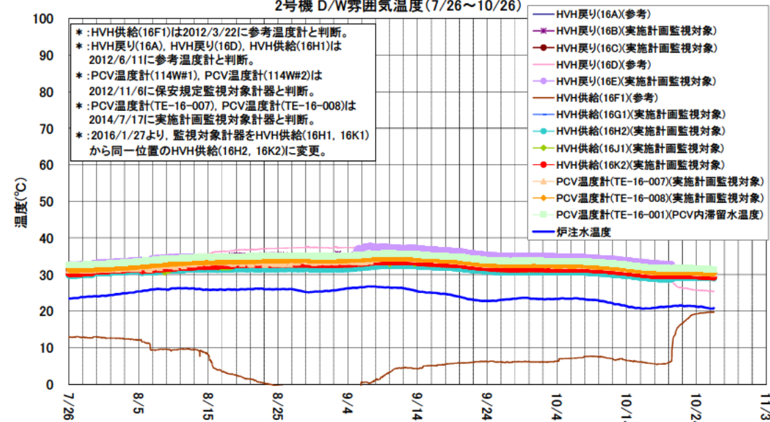
2号機 D/W雰囲気温度(7/26~10/26)
