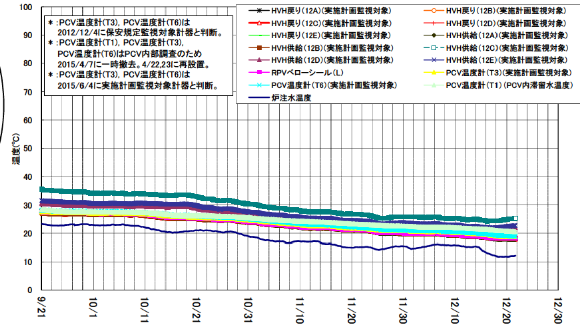
1号機 D/W雰囲気温度(9/21~12/21)
