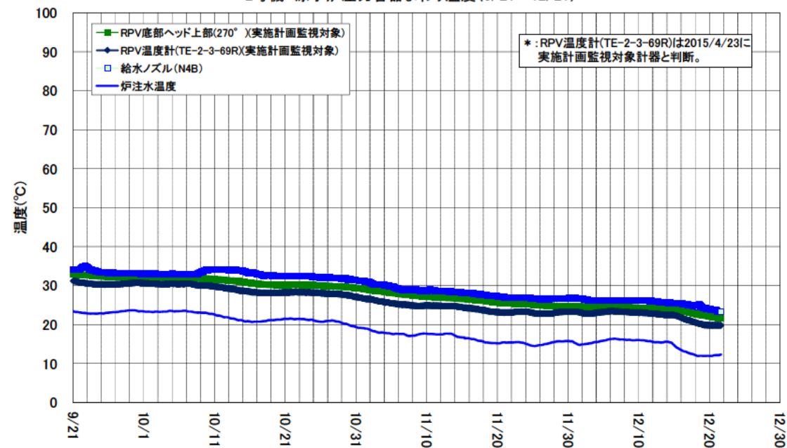
2号機 原子炉圧力容器まわり温度(9/21~12/21)
