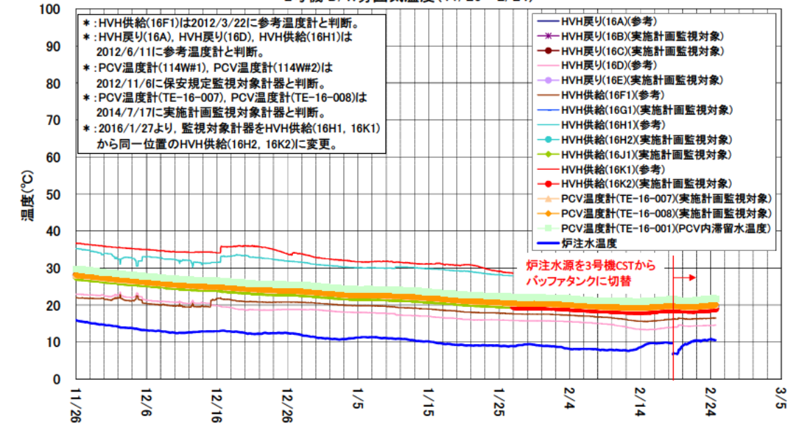
2号機 D/W雰囲気温度(11/26~2/24)
