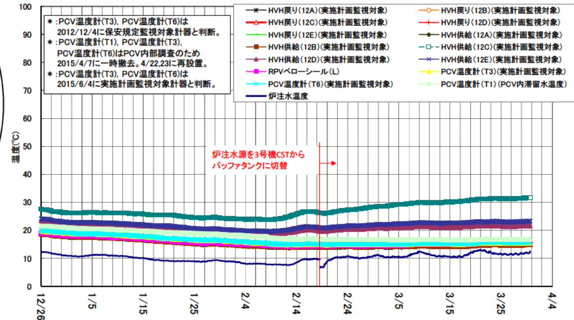
1号機 D/W雰囲気温度(12/26~3/30)
