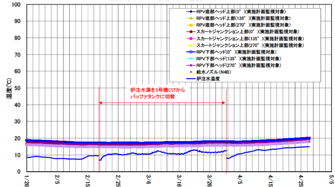
3号機 原子炉圧力容器まわり温度(1/26~4/27)
