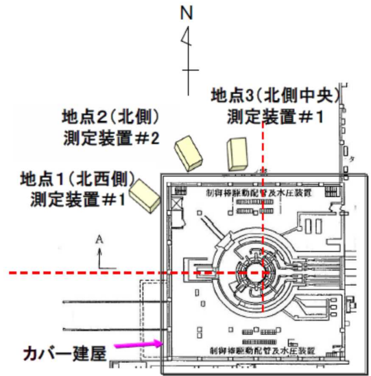
測定装置設置位置
