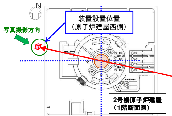
ミュオン測定装置 設置位置
