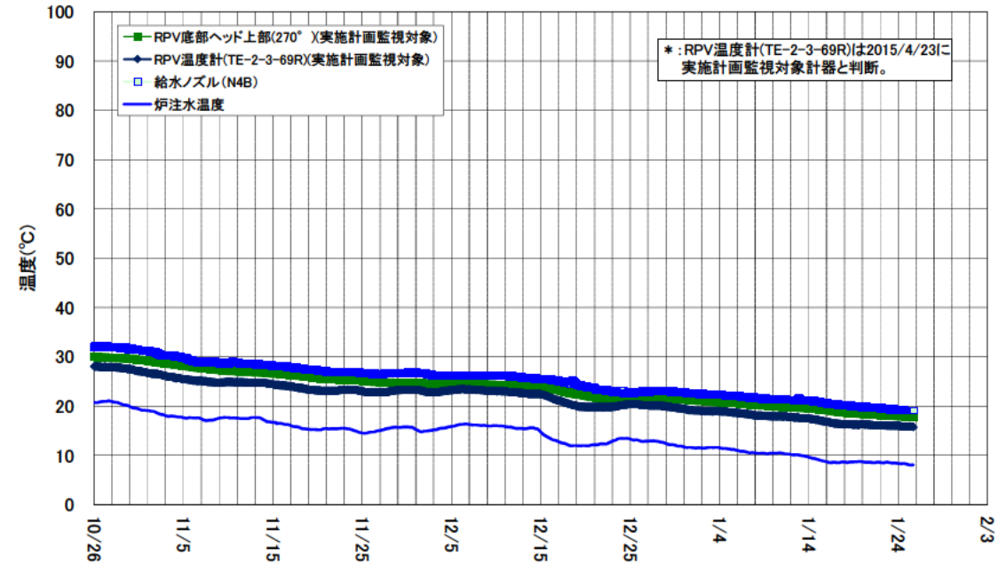
2号機 原子炉圧力容器まわり温度(10/26~1/25)
