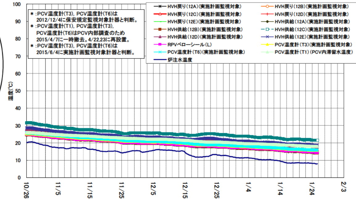
1号機 D/W雰囲気温度(10/26~1/25)
