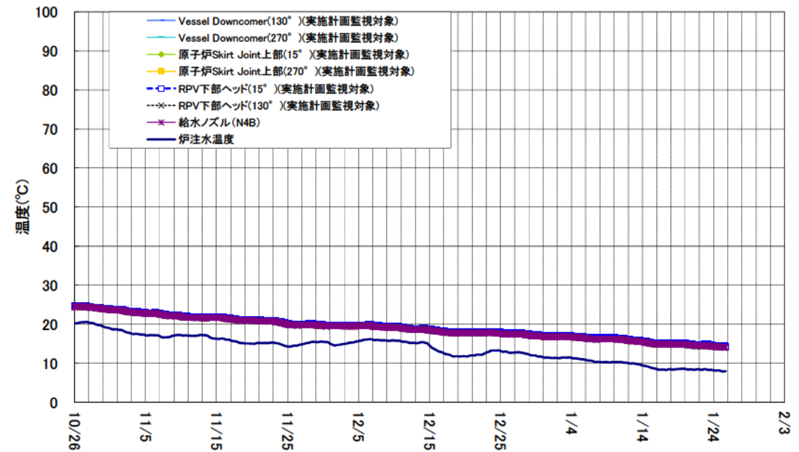
1号機 原子炉圧力容器まわり温度(10/26~1/25)
