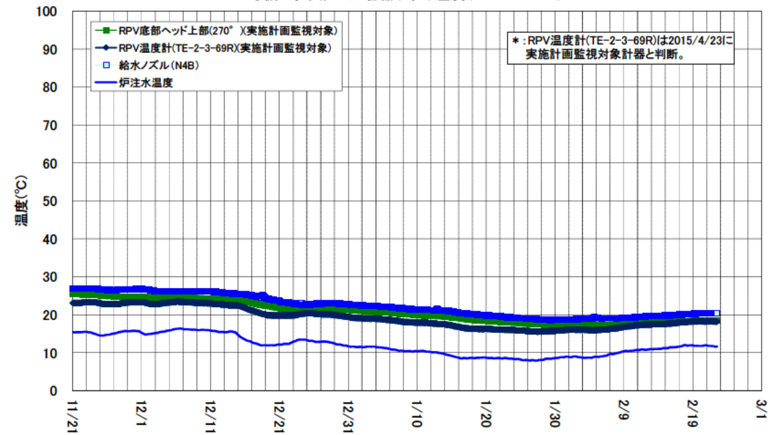
2号機 原子炉圧力容器まわり温度(11/21~2/22)
