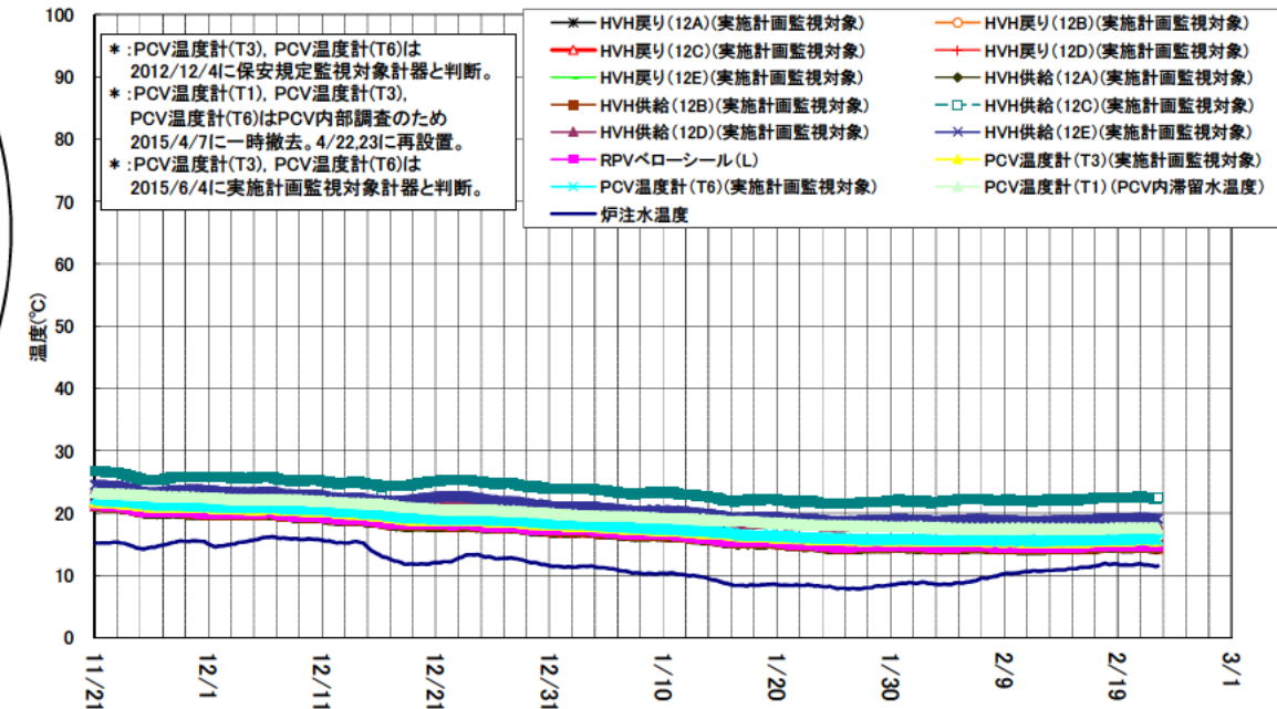
1号機 D/W雰囲気温度(11/21~2/22)
