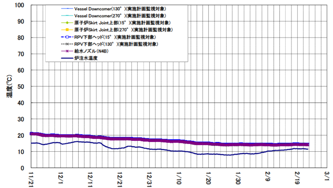
1号機 原子炉圧力容器まわり温度(11/21~2/22)
