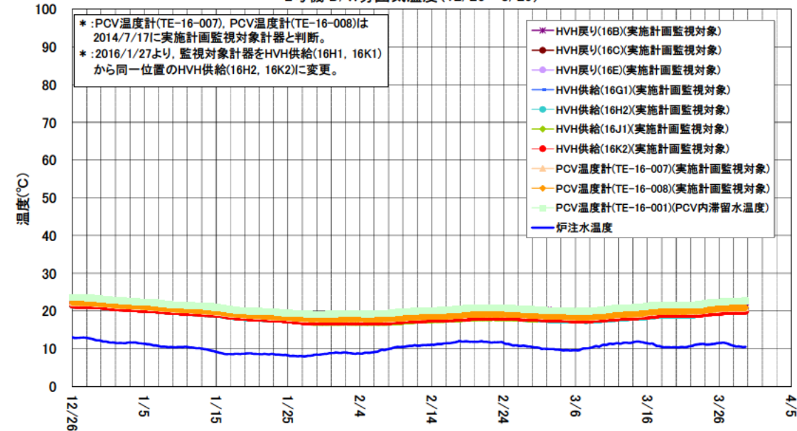
2号機 D/W雰囲気温度(12/26~3/29)
