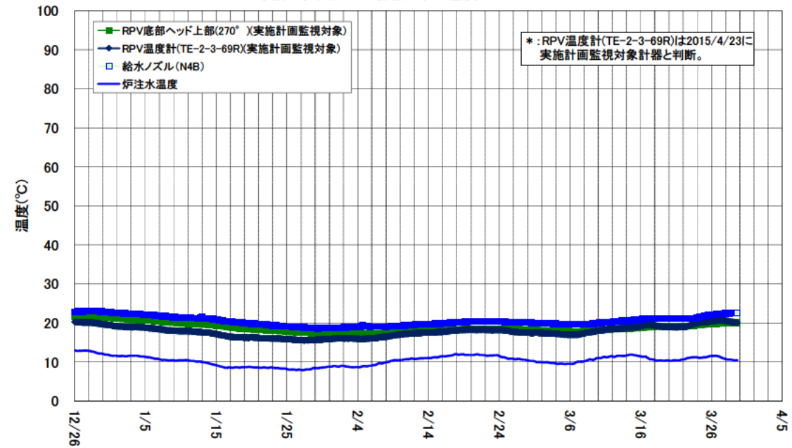
2号機 原子炉圧力容器まわり温度(12/26~3/29)
