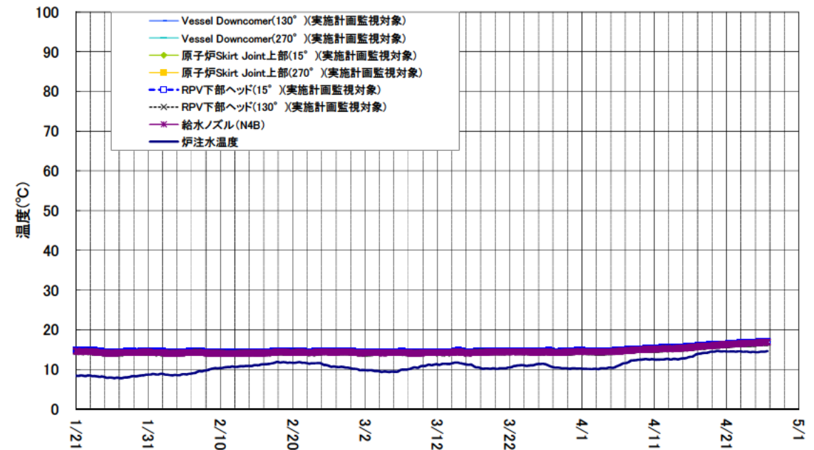
1号機 原子炉圧力容器まわり温度(1/21~4/26)
