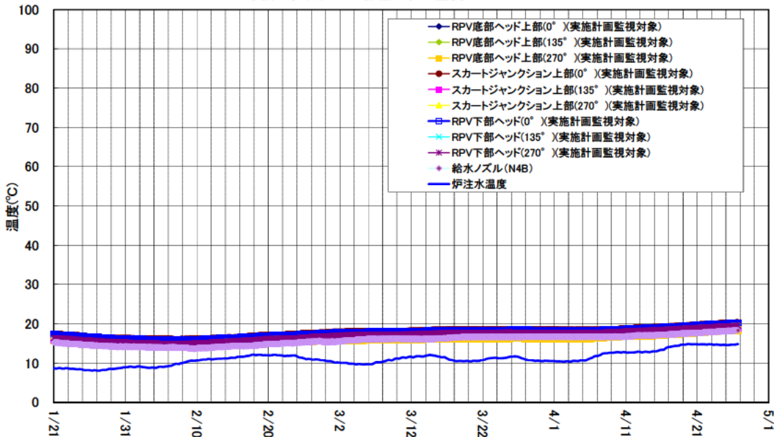
3号機 原子炉圧力容器まわり温度(1/21～4/26)
