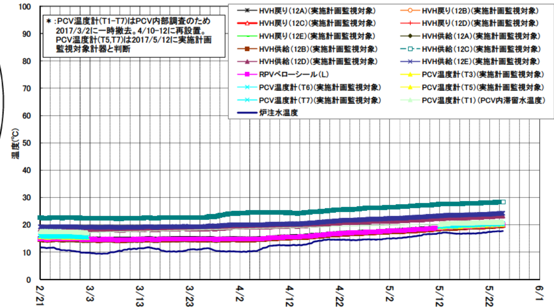
1号機 D/W雰囲気温度(2/21~5/24)
