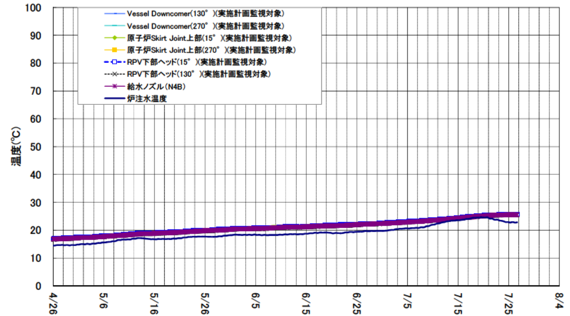
1号機 原子炉圧力容器まわり温度(4/26~7/26)
