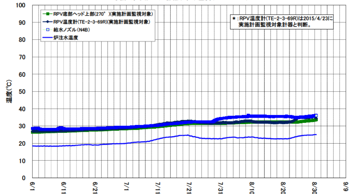
2号機 原子炉圧力容器まわり温度 (6/1～8/30)
