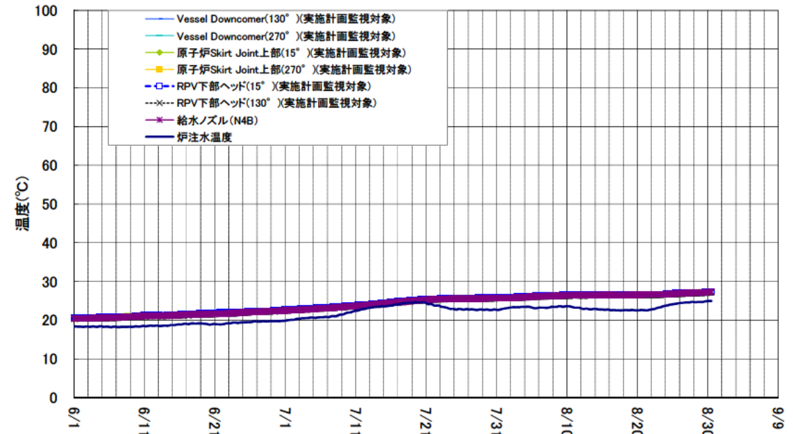
1号機 原子炉圧力容器まわり温度(6/1~8/30)
