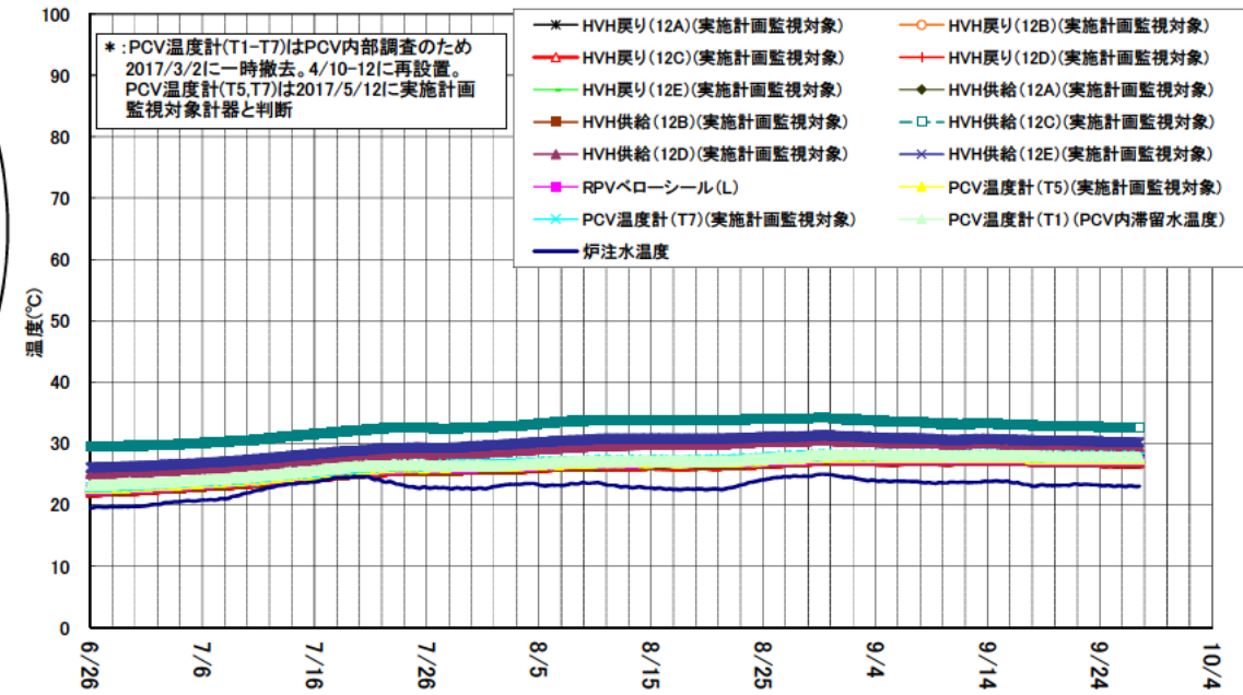
1号機 D/W雰囲気温度(6/26~9/27)
