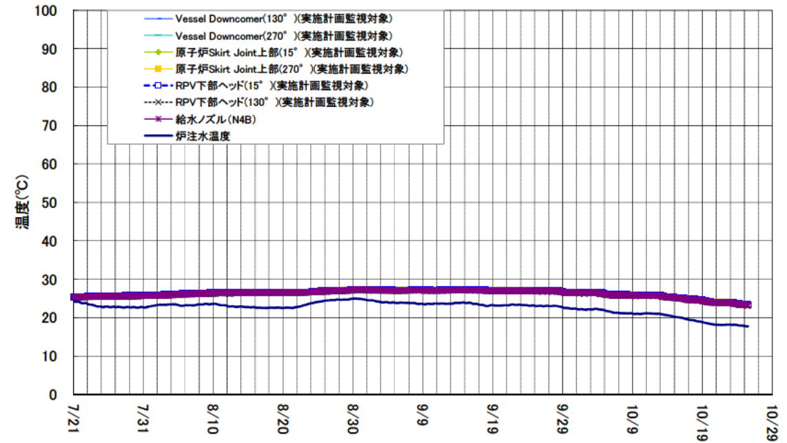
1号機 原子炉圧力容器まわり温度(7/21~10/25)
