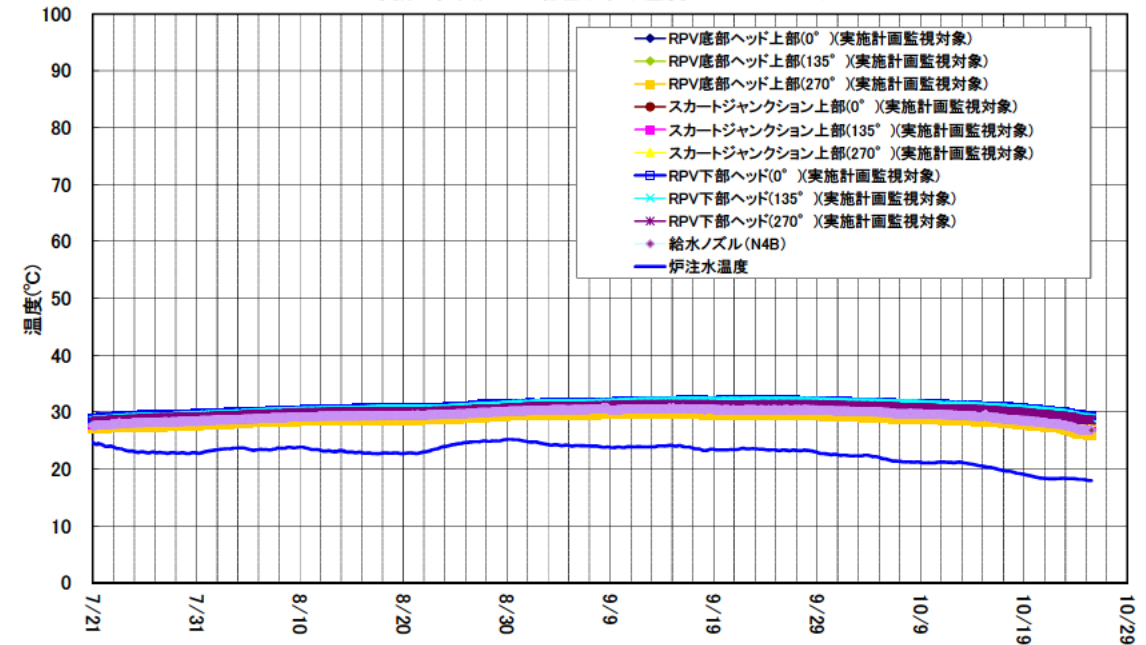
3号機 原子炉圧力容器まわり温度(7/21～10/25)
