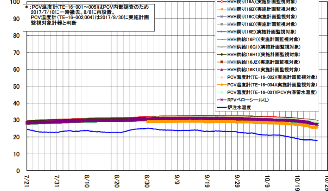
3号機 D/W雰囲気温度(7/21～10/25)
