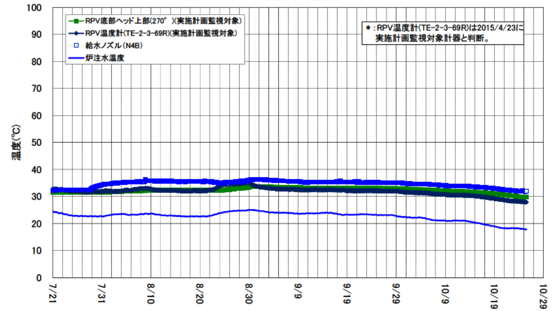
2号機 原子炉圧力容器まわり温度(7/21～10/25)
