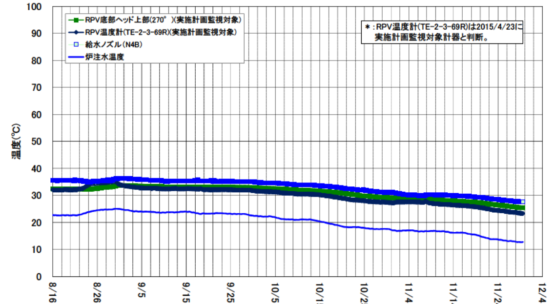
2号機 原子炉圧力容器まわり温度(8/16～11/29)
