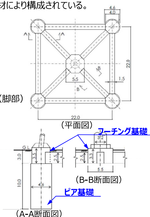
基礎部概要図
