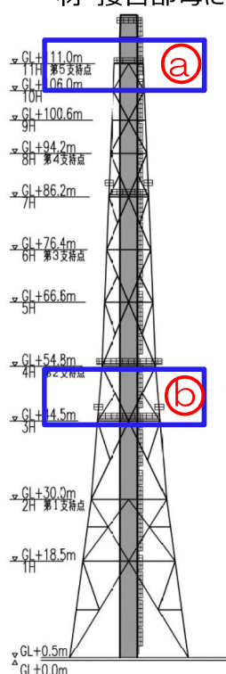
東側 立面図
