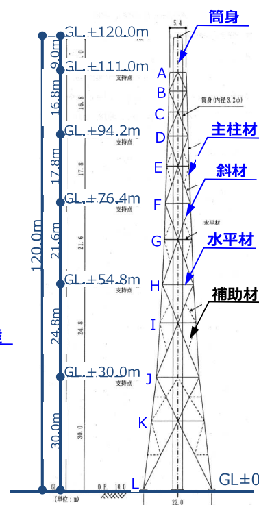
地上部概要図
