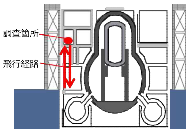
3号機原子炉建屋断面図
