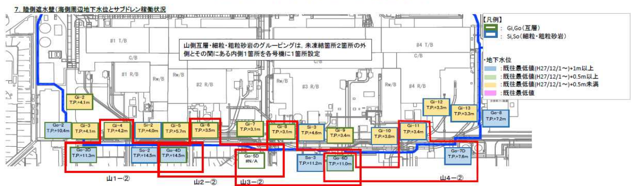
陸側遮水壁運用における監視項目（山側 互層・細粒・粗粒砂岩水頭）
