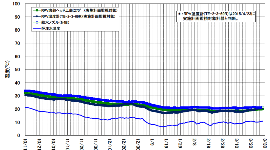
2号機 原子炉压力容器まわり温度(10/11~3/28)
