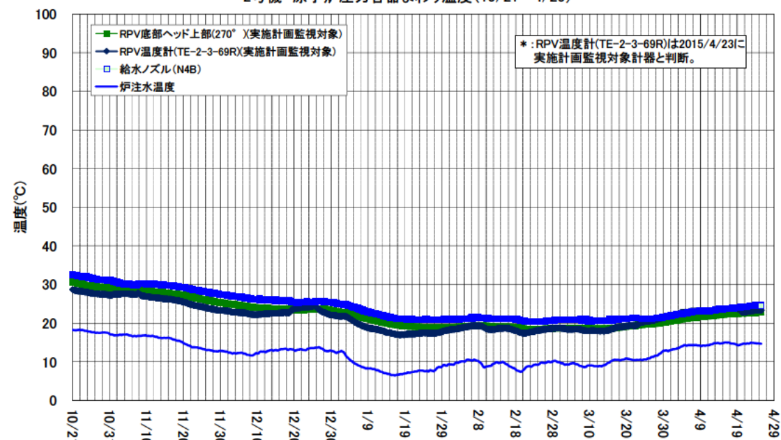
2号機 原子炉圧力容器まわり温度(10/21～4/25)
