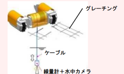
線量計、カメラ吊り降ろしイメージ
